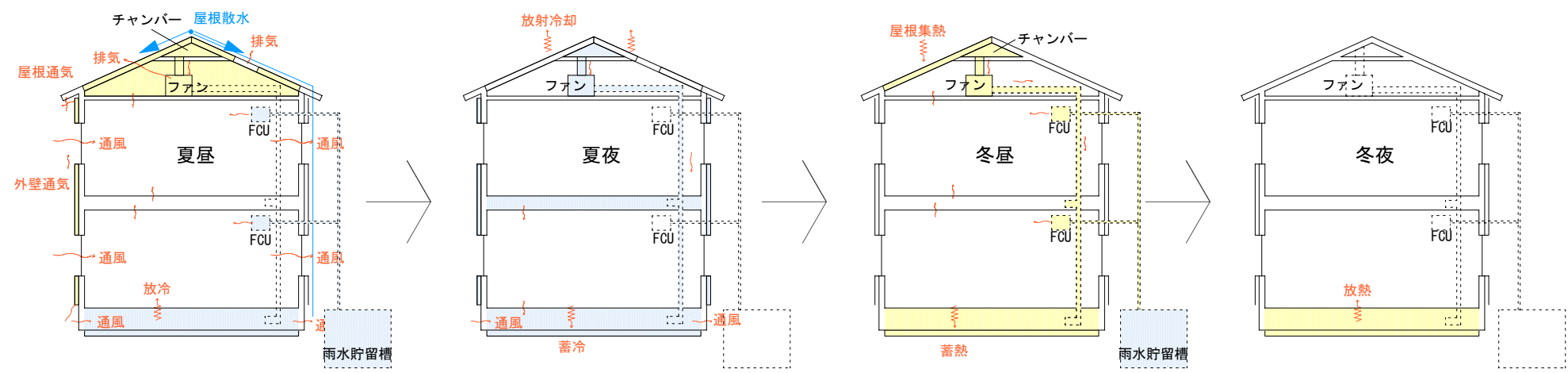
空気循環システム図
